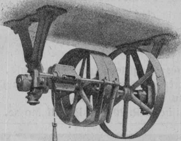
Riemenrucker Typ Clus, mit nur einem Zugseil
