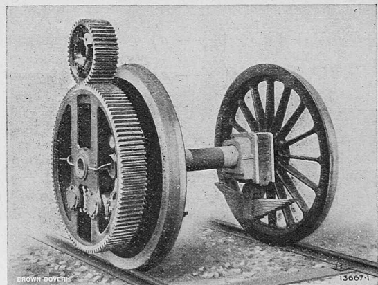
Abb. 9. Triebachsatz mit Zahnradgetriebe.
