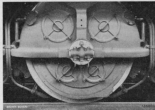
Abb. 12. Zahnrad-Verschaltung mit achsial aufgebauter Öelumlaufpumpe.
