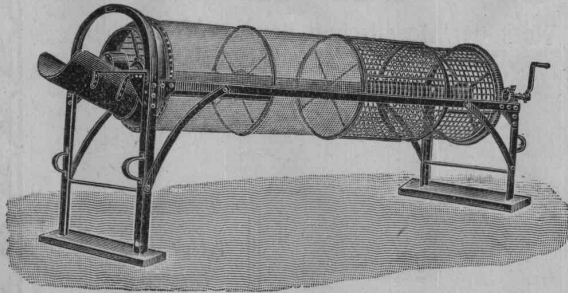
Sortiertrommel
