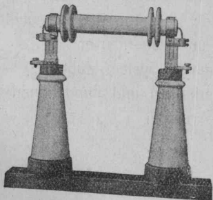
Hochspannungs-Sicherung, Type 5k20
