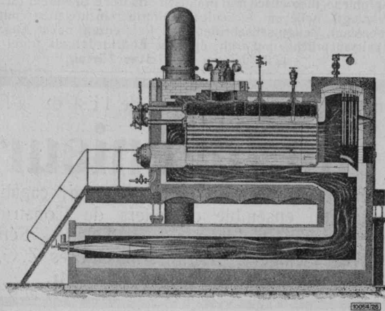
Horizontaler Abhitze-kessel verbunden mit einem Glühofen, in der Schmiede der Schweiz. Industriegesellschaft Neuhausen
