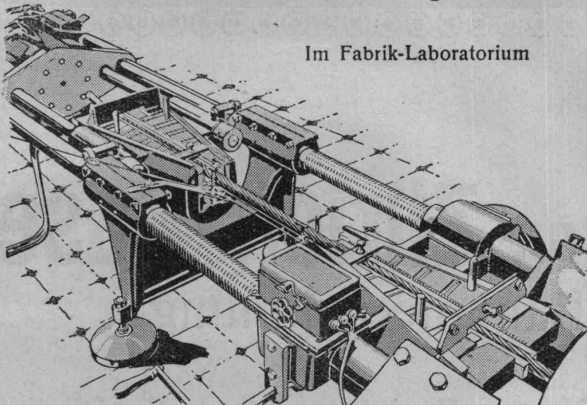
Drahtseil-Zerreiss-Versuch
