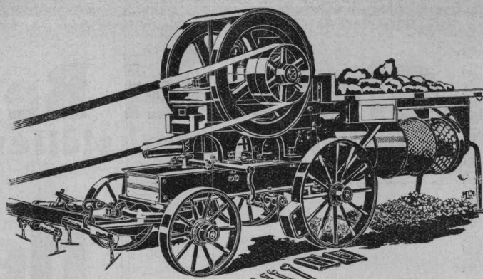
Steinbrechanlage mit Sortierzylinder.
