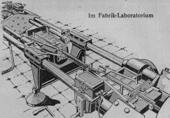
Drahtseil-Zerreiss-Versuch
