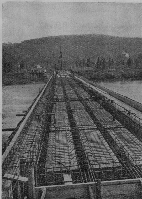
Vom Bau der Eisenbahnbrücke über die Aare bei Döttingen-Klingnau. Armierung der Fahrbahnplatte.
