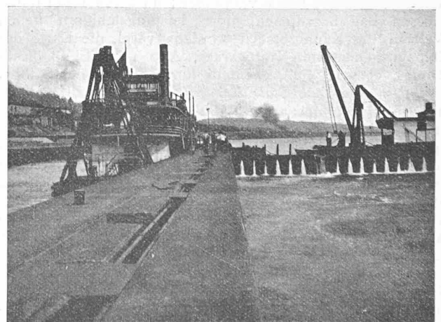
Abb. 4. Schleuse und Klappenwehr im kanalisiertem Ohio. Schleusen-Länge 183 m, Breite 33,6 m, Drempeeltiefe 3,35 m.
