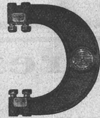
Nachstellbare Rachenlehre
