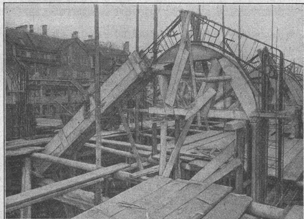
Shaw-Konstruktionen einer Seidenfärberei in Zürich.
