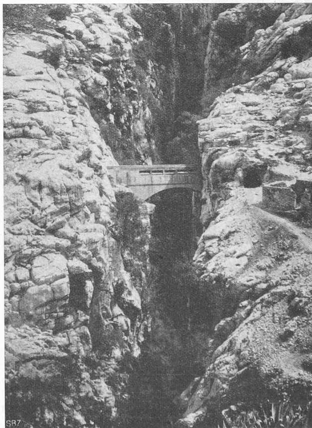
Fig. 13. Vue d'amont de l'aqueduc sur le Guadiaro.
