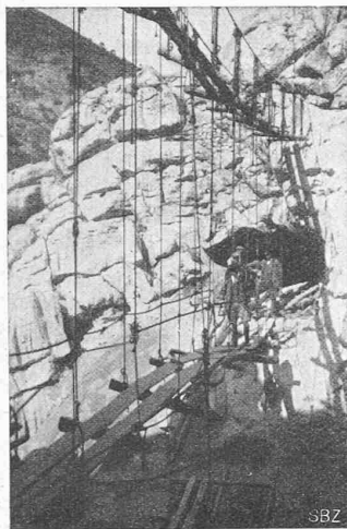
Fig. 16. Passerelle suspendue ayant servi à la construction du cintre pour l'aqueduc.
