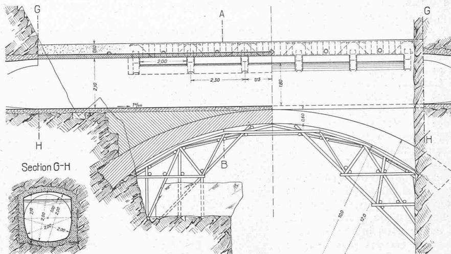
Fig. 14. Aqueduc avec déversoir, pour la galerie d'aménée, dans la gorge de Buitreras. — Vue d'amont et coupe en long, et section du raccord à la galerie. — Echelle 1 : 150.
