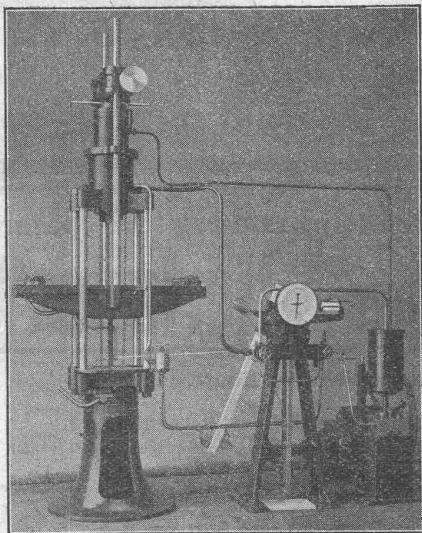
30 tons Zerreissmaschine
