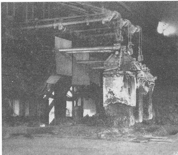
Abb. 5. Frühere Elektroden der Ofenanlage in Anniston.
