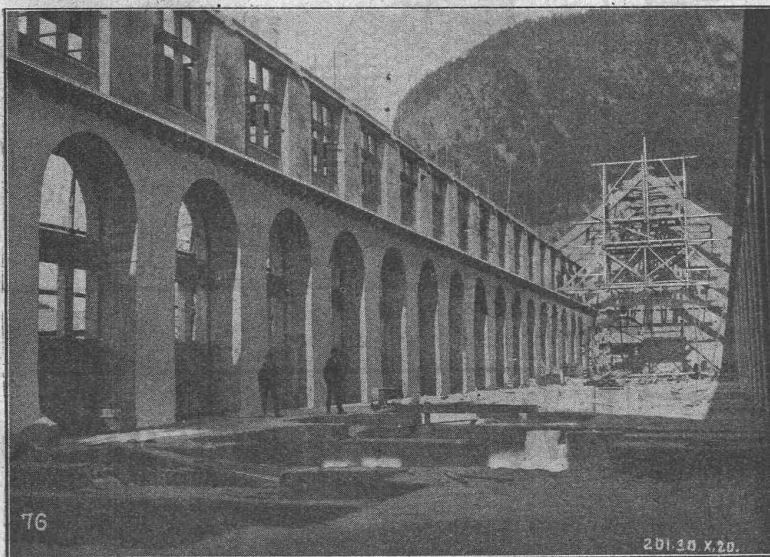
Maschinenhaus des Kraftwerkes Amsteg SBB. Bauzustand Ende Oktober 1920.
