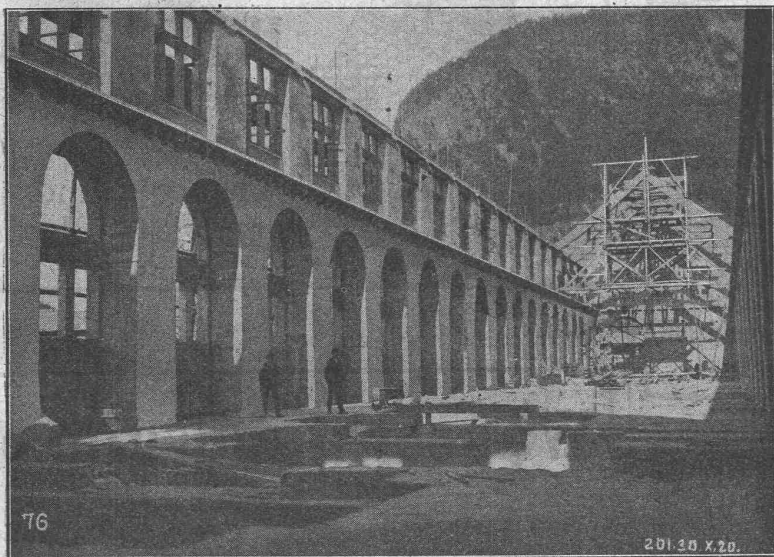
Maschinenhaus des Kraftwerkes Amsteg SBB. Bauzustand Ende Oktober 1920.
