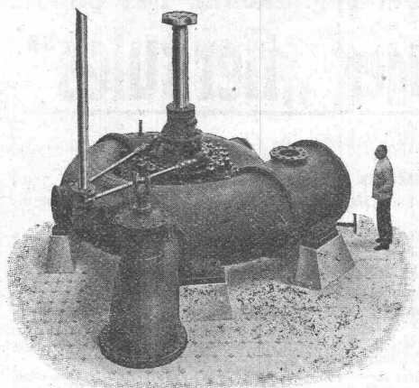
Turbine spirale de 6000 HP sous 105 m de chute pour l'Usine de la Jagne des Entreprises Elec- triques Fribourgeoises.
