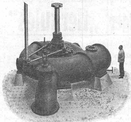
Turbine spirale de 6000 HP sous 105 m de chute pour l'Usine de la Jogne des Entreprises Electriques Fribourgeoises.
