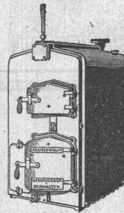
Zoller- Warmwasserkessel.
