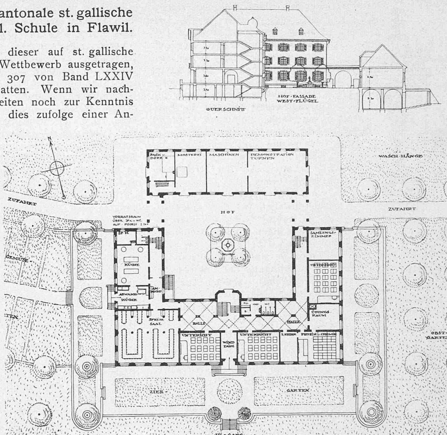
I. Preis (5000 Fr.), Entwurf Nr. 10. — Grundriss vom Erdgeschoss und Querschnitt. — 1:800.
