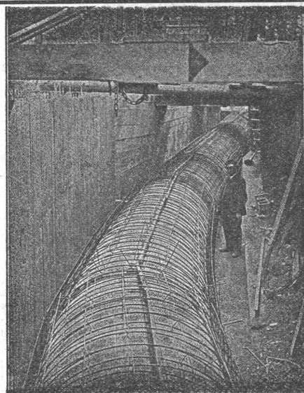
Druckrohr im Eisenbeton von 2 m Durchmesser der Wasserkraftanlage Stöcklin & Cie., Basel, 1916/17.
