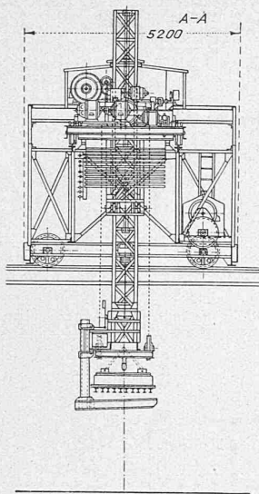
Abb. 3. Seitenansicht der Laufkatze mit Hubvorrichtung. Masstab 1 : 150.
