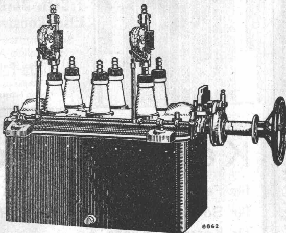
Dreipoliger Oelschalter mit aufgebauten Hauptstromzeitrelais.
