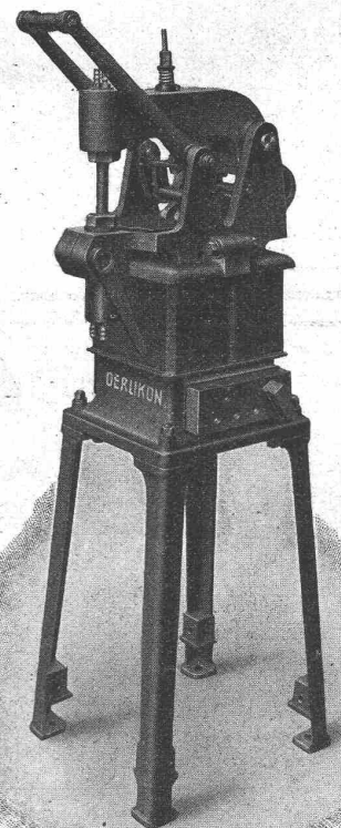
Maschine zum Erwärmen von 40–50 Niete (Durchmesser bis 25 mm, Schaftlänge bis 120 mm) pro Stunde. Stromverbrauch 8–10 kW.
