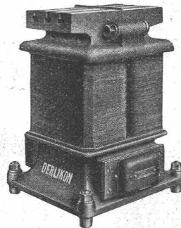
Transformator ohne Ausrüstung, mit genutetem Aufspanntisch zum Befestigen der verschiedenen Vorrichtungen, z. B. für Nahtschweißung, oder für Stumpfschweißung, Schweißung von Rohrnähten, für das Erwärmen von Niete u. s. f.
