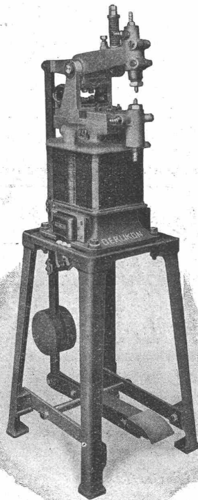
Transformator mit Punktschweisseinrichtung. Nach Auswechslung der Elektroden können Niete bis 16 mm Schaftdurchmesser nietbereit erwärmt werden.
