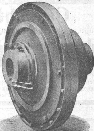
Elektromagnetische Reibungskupplung Patent.
