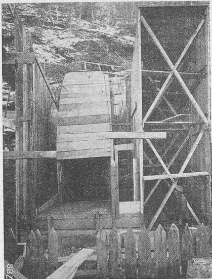
Abb. 14. Ventilatoren-Verschaltung.
