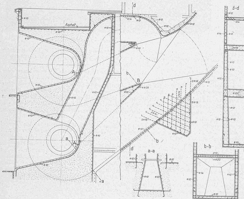
Abb. 11. Vertikal-Schnitte des Ventilatoreng Gebäudes. — Masstab 1:200.
