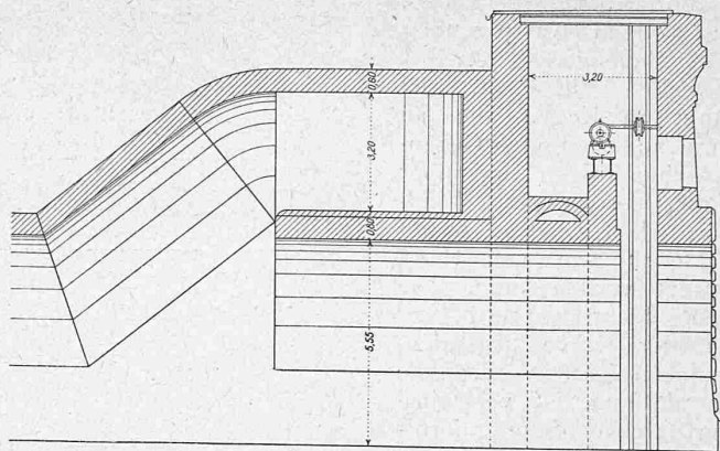
Abb. 17. Einmündung („Pfeife“) des Luftkanals in den Tunnel, Längsschnitt (rechts das Tunnelportal). — 1:200.
