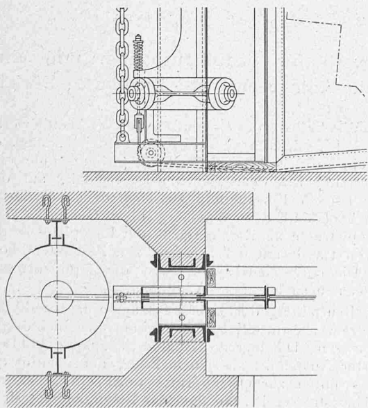
Abb. 19. Rahmenfuss zum Abschluss-Vorhang, darunter: Horizontalschnitt. — Masstab 1 : 30.
