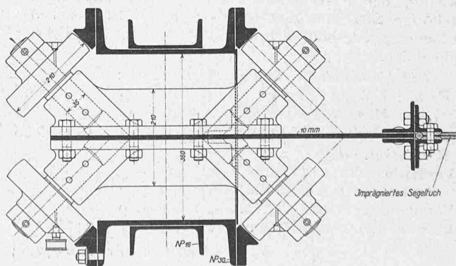
Abb. 20. Führungsrollen des Vorhang-Rahmens. — 1 : 10.
