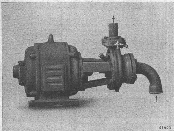
Hauswasserpumpe bestehend aus einer einstufigen Sulzer-Zentrifugalpumpe, direkt an einen BBC-Drehphasenmotor angebaut.
