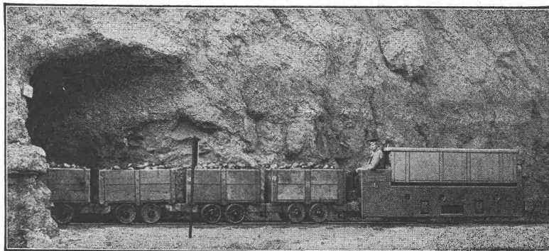
Grubenbahn Gr. Bülten, mit abrollbarer Batterie
