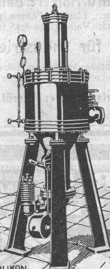
Elektroden-Dampfzeuger, Syst. Revel, 500 kW
