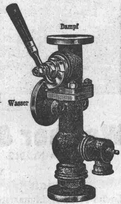
zum Kessel
