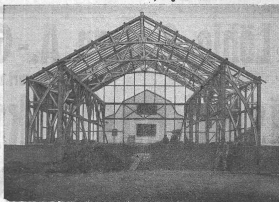
Zweigelenkbinder mit Krahnbahn in „Holzfachwerk“ Waagenfabrik J. Studer in Olten
