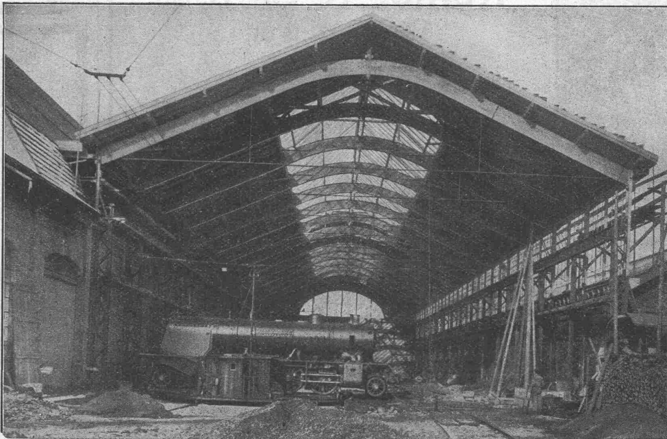
Montagehalle der Schweiz. Lokomotiv- und Maschinenfabrik Winterthur. Spannweite der Hetzerbinder 24 \frac{1}{2} m.
