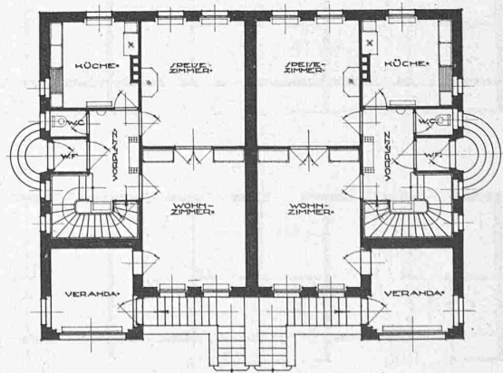
Abb. 4. Grundriss vom Erdgeschoss.
