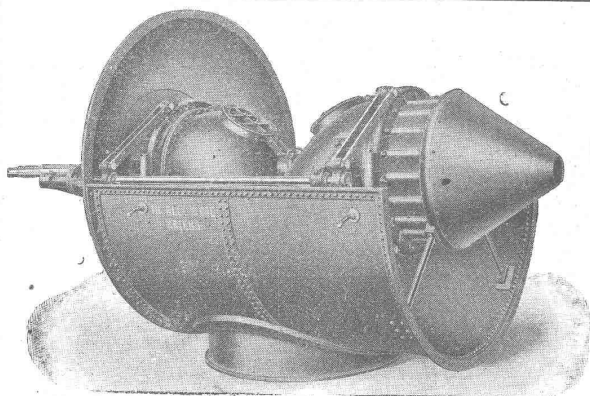
Zwillingfrancisturbine in geschlossenem Blechkessel.
