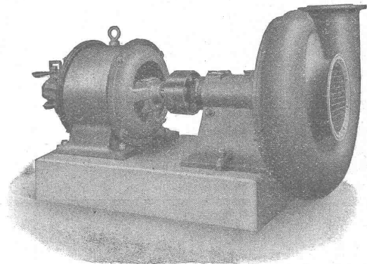
Einstufiger Hochdruck-Zentrifugalventilator
