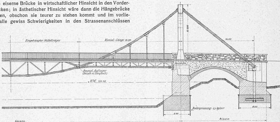
Angekaufter Entwurf Nr. 3. — Verfasser: Ingenieur A. Walther, Direktor der Firma W. Koch & Cie. in Zürich, mit Architekt Rich. v. Muralt in Zürich.
