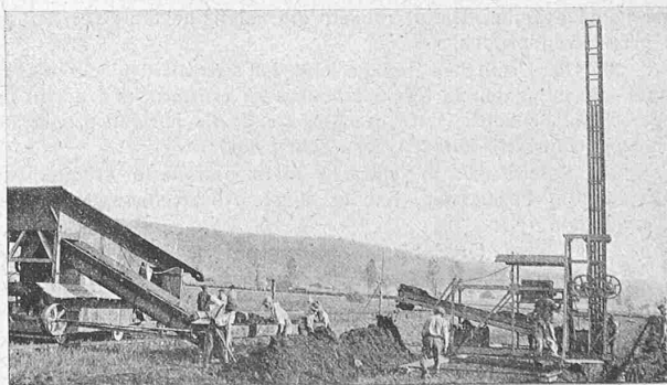
Torstechmaschine (rechts) und Verarbeitungsmaschine in Betrieb.
