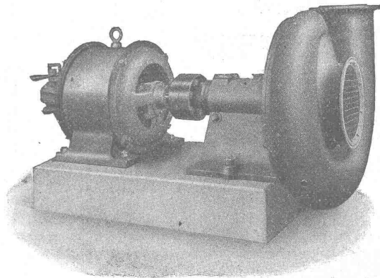
Einstufiger Hochdruck-Zentrifugalventilator
