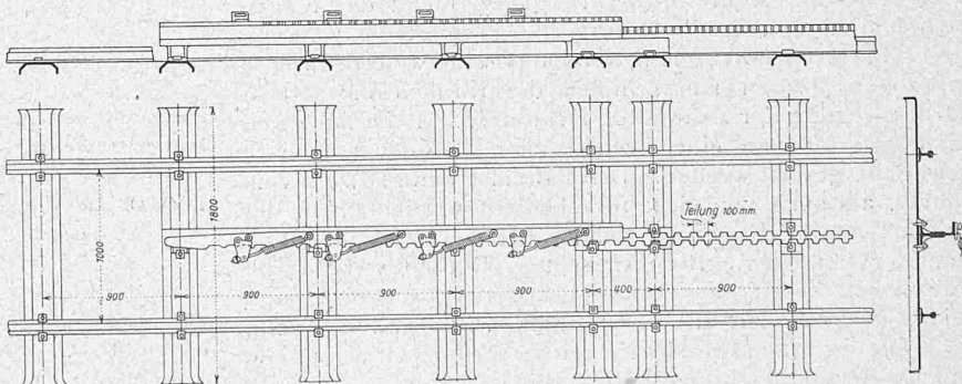
Abb. 6. Zahnstangen-Einfahrt. — Masstab 1 : 50.
