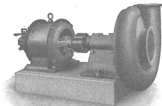
Einstufiger Hochdruck-Zentrifugalventilator
