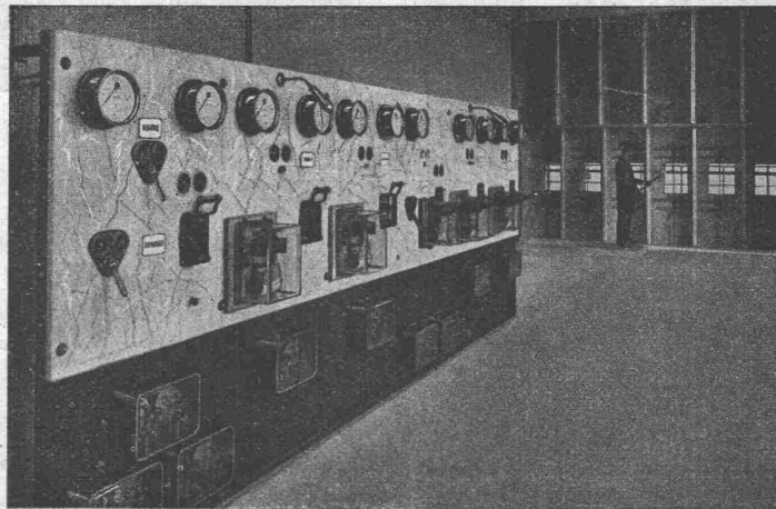
Tafel und Zellenbau in einer Transformatorstation des 65 000 Volt-Verteilungsnetzes Nancy.
