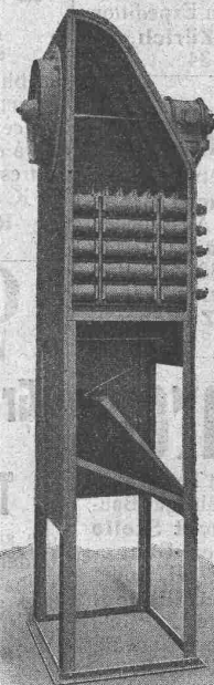
Sendric-Fabrik-Heizapparat mit Frischluft-Beimischklappe. (Seltenwand weggenommen). Leistung: 50000 WE/Std. Kraftverbrauch: 0,5 PS.
