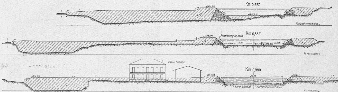
Abb. 3 bis 7. Querprofile der Sihlverlegung. — Masstab 1 : 1000.
