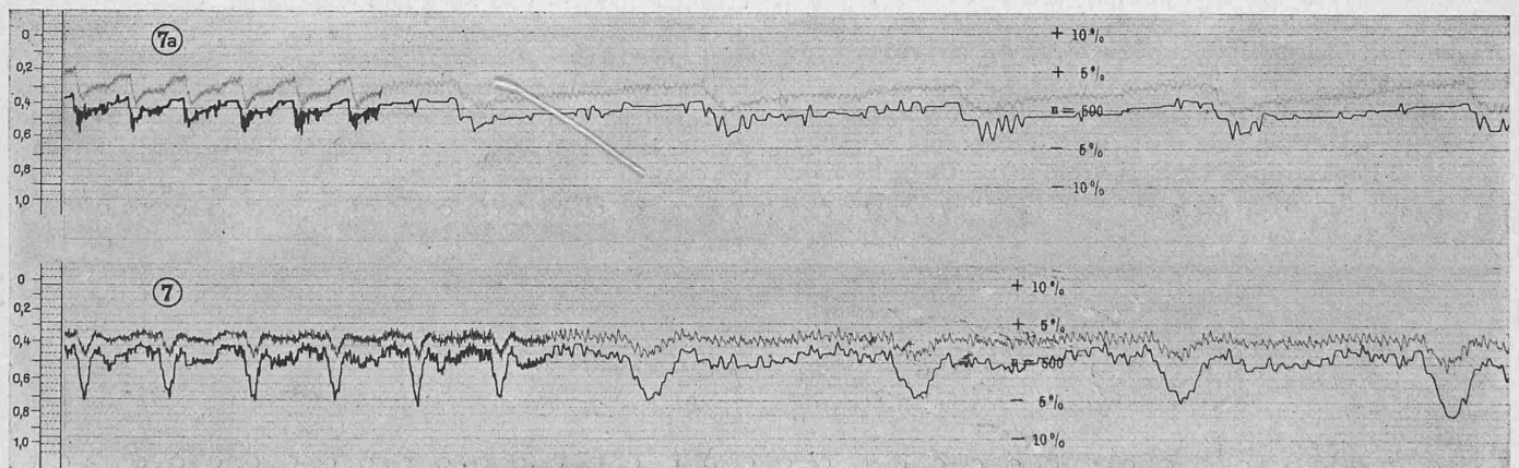
Abb. 13. Betrieb von einem Selfaktor mit der Turbine allein. — Zeitmasstäbe: Oben 0,5, später 2,5 mm = 1 sek; unten 0,65, später 2,5 mm = 1 sek.
