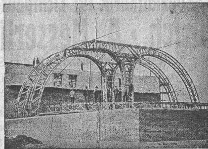
Bogenkonstruktion in Holz, System Meltzer
