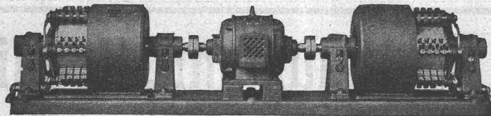
Phasenkompensationsaggregat zur Verbesserung des Leistungsfaktors eines 760 KW-Asynchrongenerators von 0,82 auf 1. Leistung des Antriebmotors 1,5 KW.
