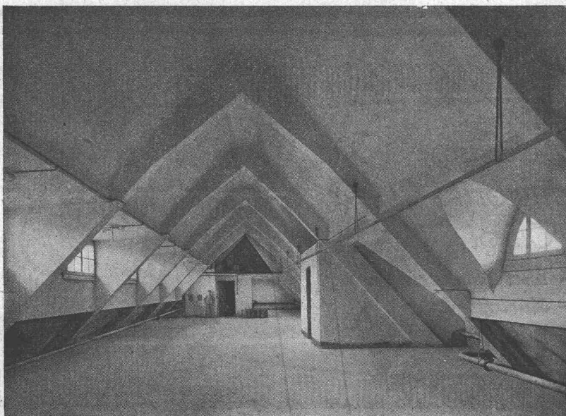
Bankgebäude in Zürich — Dachstuhl in Eisenbeton
