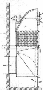
Sendric-Fabrik-Heizapparat mit Frischluftzuführung für Leistungen bis 360 000 WE pro Apparat und Stunde.
