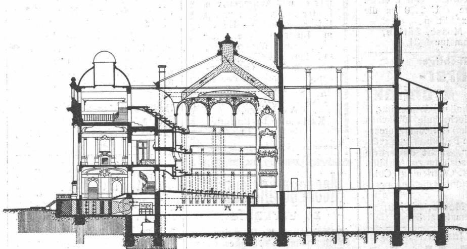
Abb. 1 Platzbedarf einer Sendric-Anlage
