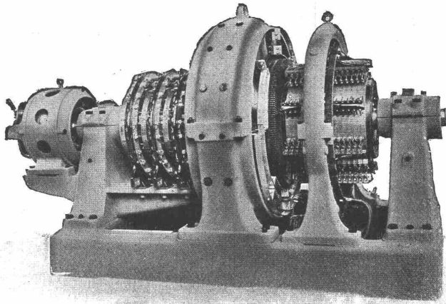
Einanker-Umformer.
