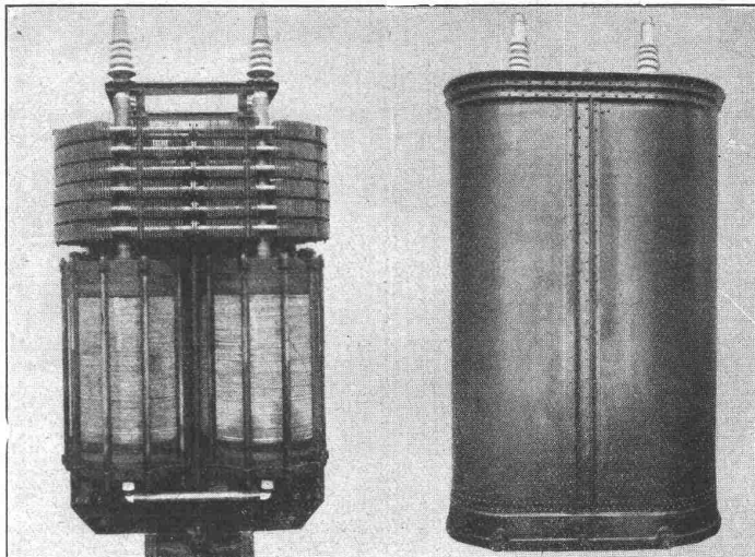
Einphasen-Wechselstrom-Transformator von 2400 kVA, 6000/60 000 Volt, 16 \frac{2}{3} Per.
