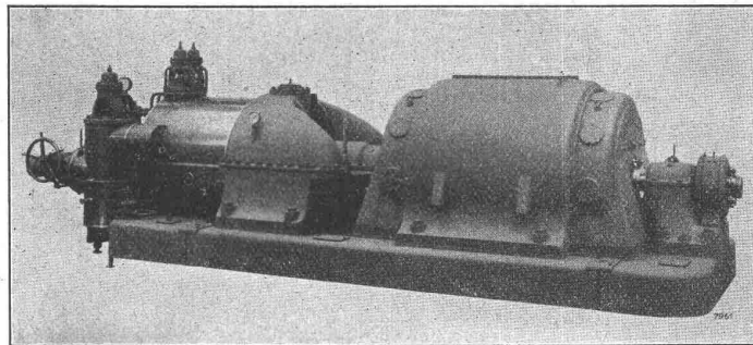
Drenstrom-Turboaggregat, Normalleistung 5000 kW, 3000 Umdr./Min.
