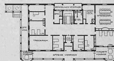
ERDGESCHOSS - MÄNNERABTEILUNG
