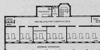
OBERGESCHOSS
