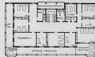
OBERGESCHOSS - FRAUENABTEILUNG
