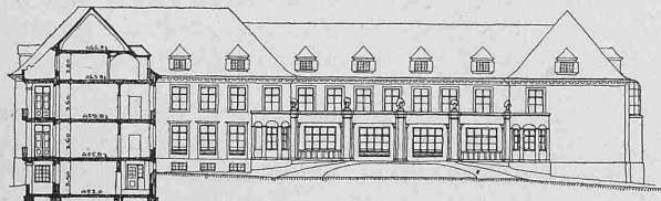
Schnitt und Ansicht des Nordflügels mit Anfahrt.
