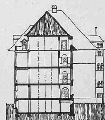
Schnitt 1 : 800.
