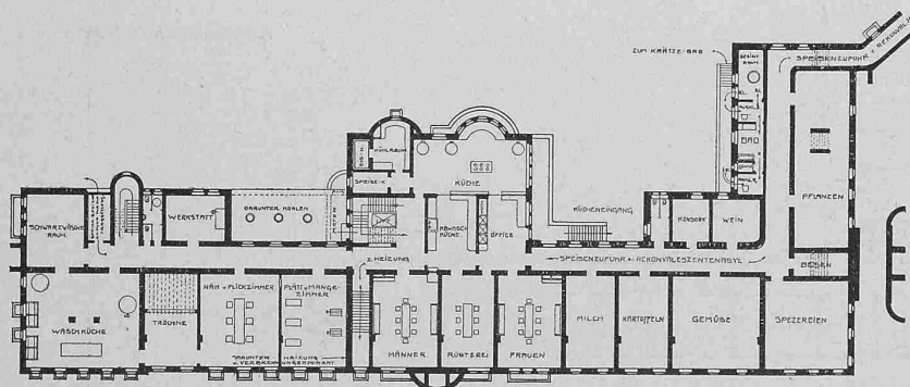
Entwurf Nr. 23. Grundrisse des Hauptgebäudes.
