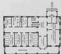
Rekonvaleszenten-Heim 1:800.
