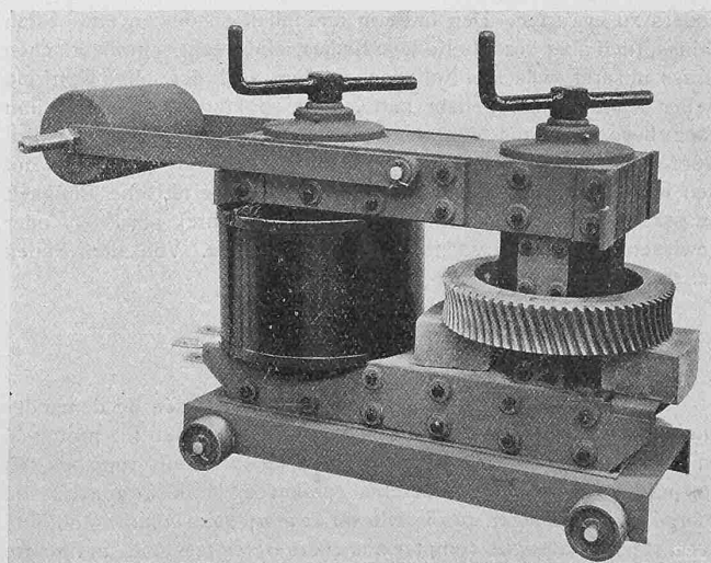
Abb. 2. Geschlossene Stellung.
