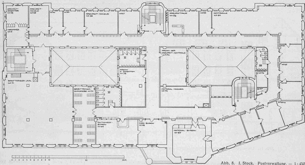
Abb. 8. 1. Stock. Postverwaltung. — 1:450.
