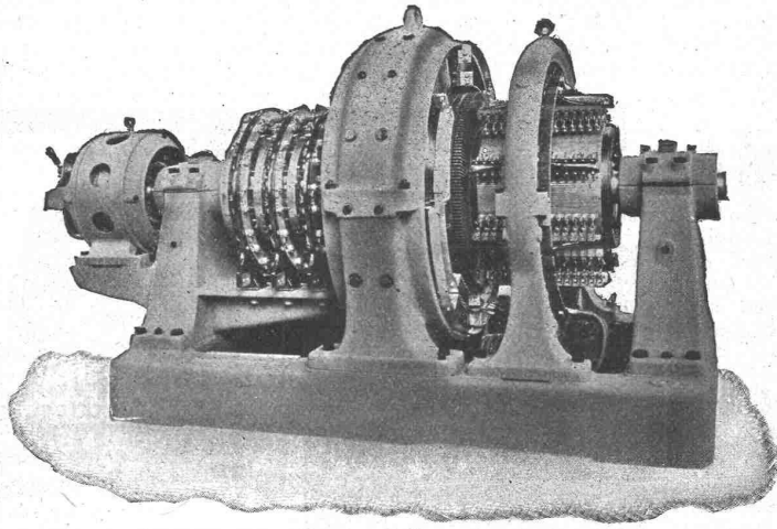
Einanker-Umformer.
